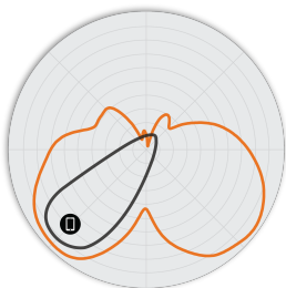
图 5. R760 2.4GHz 俯仰 天线模式
