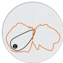
图 6. R760 5GHz 俯仰 天线模式
