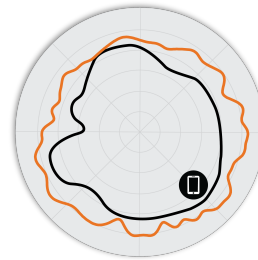
图 7. R760 6GHz 俯仰 天线模式
