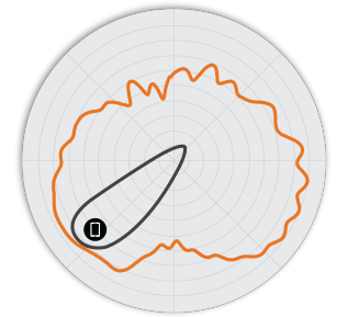
Figure 5. Diagrammes d'antennes Élévation R350 5 GHz
