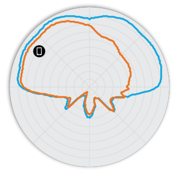
图 5. R850 5GHz 俯仰 天线模式
