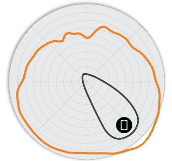
Figure 5. Diagrammes d'antennes Élévation R650 5 GHz
