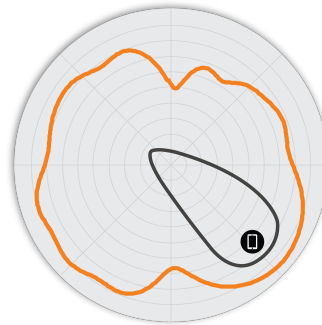
Figure 4. Diagrammes d'antennes Élévation R650 2,4 GHz
